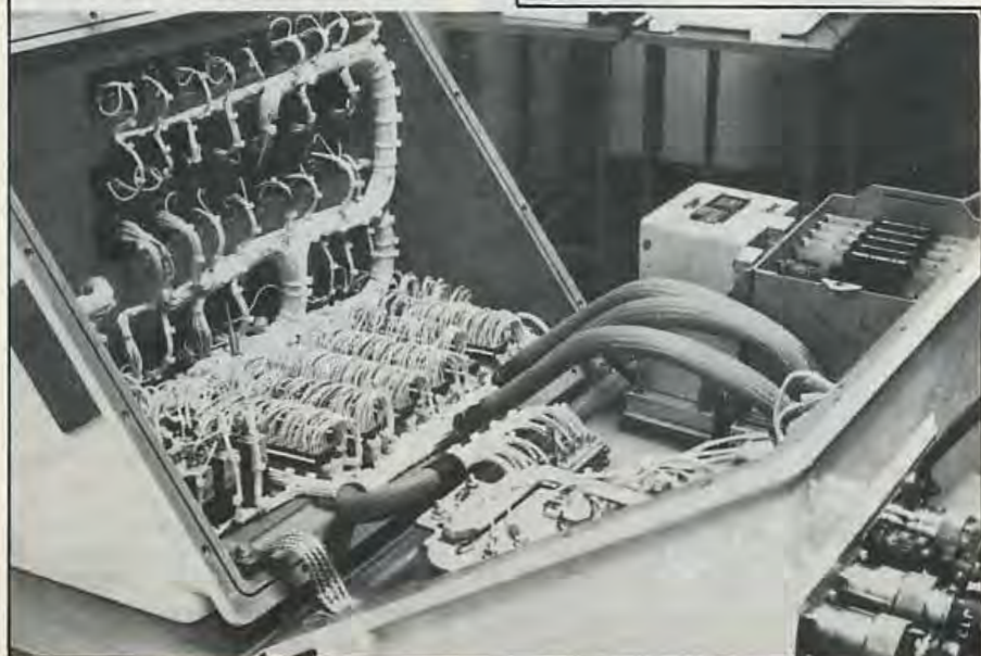
B1 complète (Tourelle T 105 MI). 190 mesures effectuées en 14 mm.
